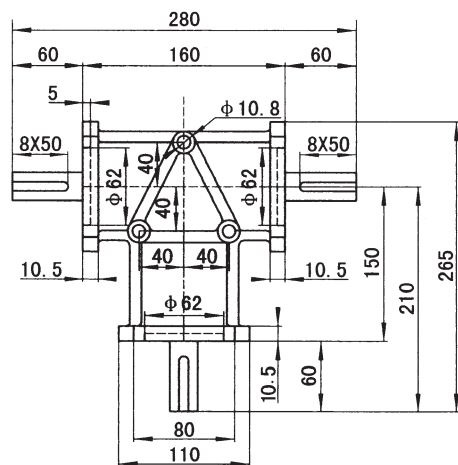
ARA4外型尺寸图
