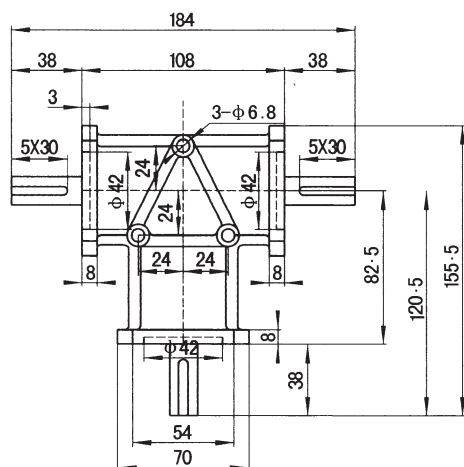
ARA1外型尺寸图
