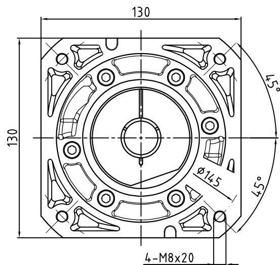
输入端(Input)
