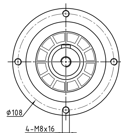
输出端(Output)
